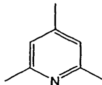
sym -Collidine Bp 172 °C pK a = 7.43
